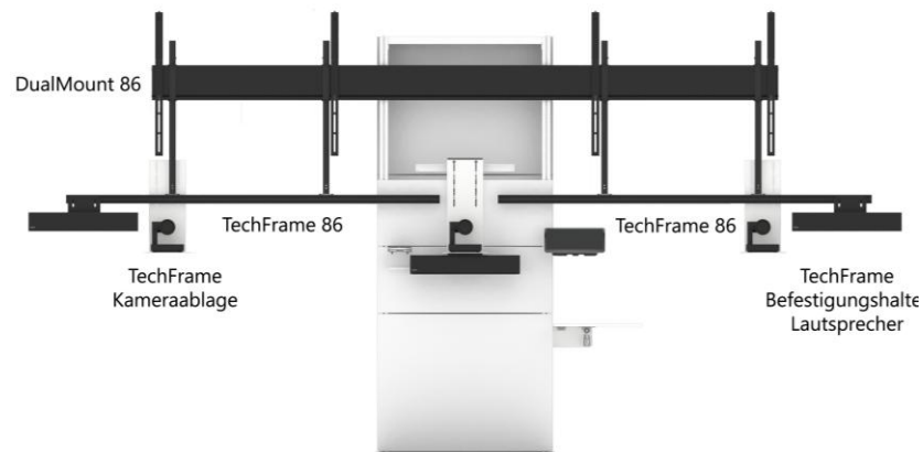
Beispiel: Mediastele mit DualMount, TechFrame, Kamera- und Soundbarablagen
